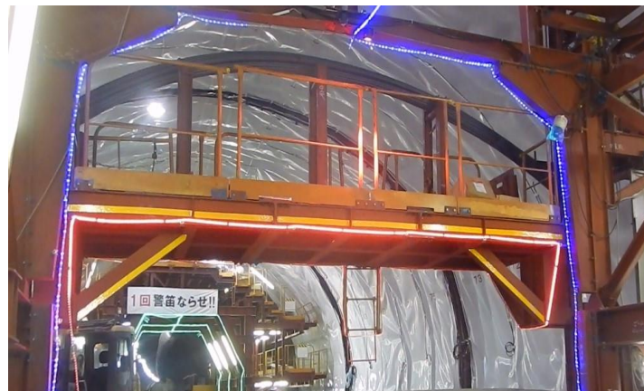
主筋搬入姿 (台車の内側から見る)
